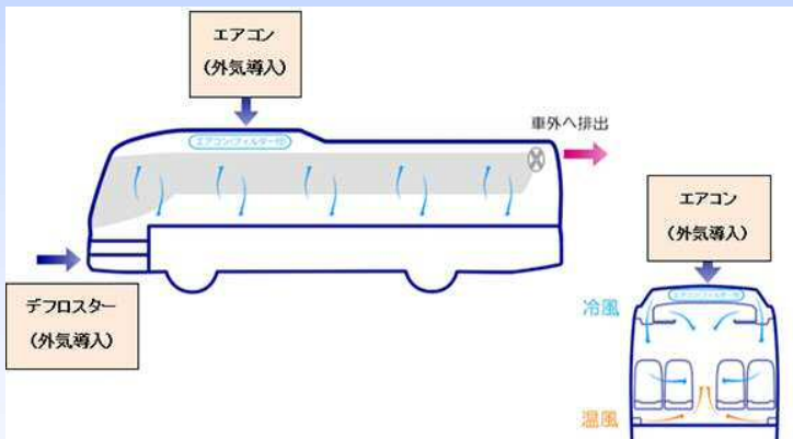
外気導入システム
